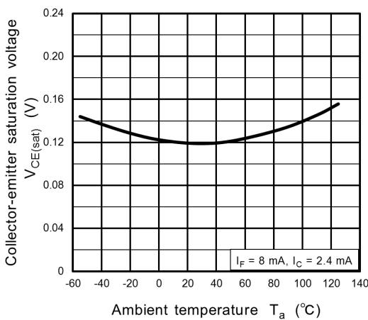
Fig. 11.10 V_{CE(sat)} - T_a
