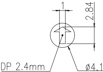
ACTUATOR
