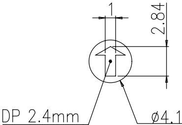
ACTUATOR
