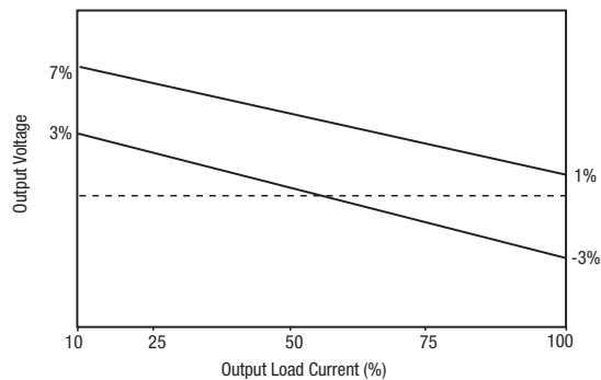
CRE1S0505S3C
