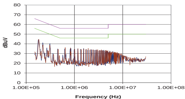
CRE1S0505S3C
