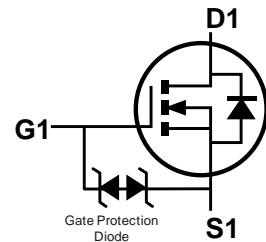
Q1 N-CHANNEL
