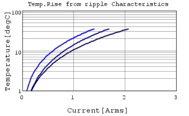
GRT155R61E474KE01 Temp.rise — 200kHz —
