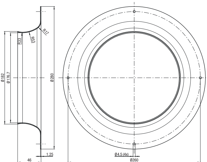
Fan size 280:
