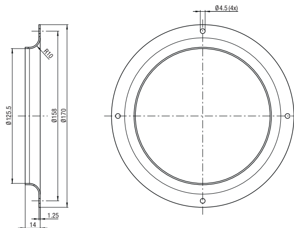
Fan size 175 / 190:
