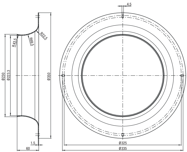
Fan size 355:
