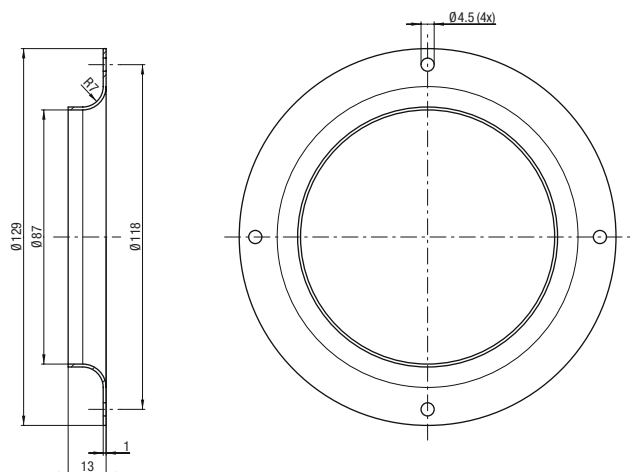
Fan size 133:
