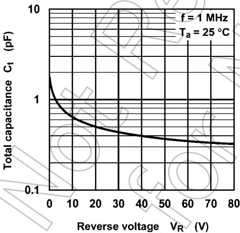
Fig. 8.3 C t - V R
