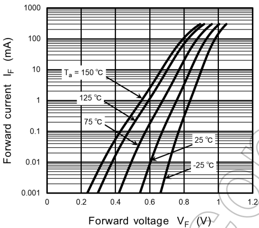
Fig. 8.1 I F - V F
