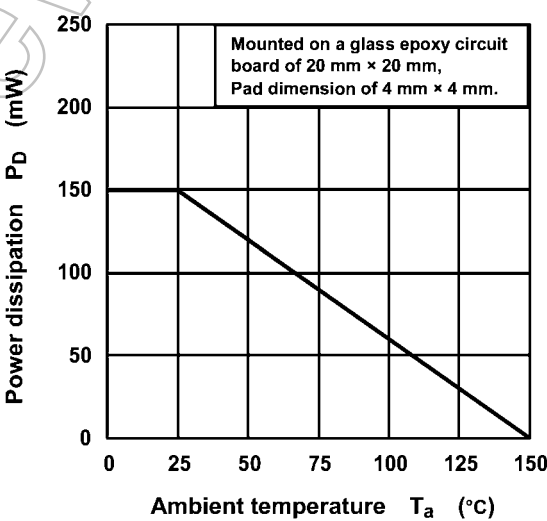
Fig. 8.4 P D - T a
