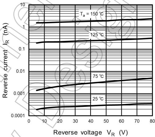
Fig. 8.2 I R - V R
