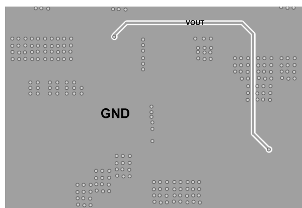
Bottom Layer
