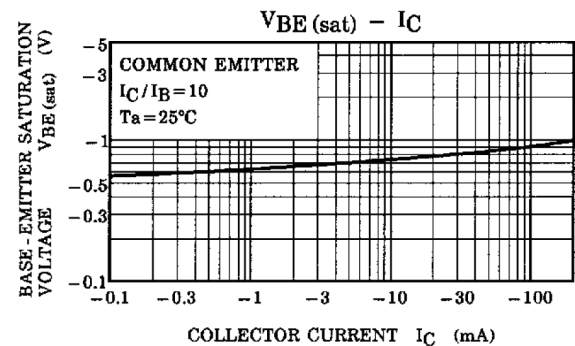
Fig. 8.4 V_{BE(sat)} - I_C
