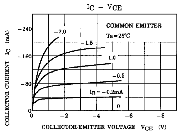
Fig. 8.1 I_C - V_{CE}
