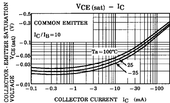
Fig. 8.3 V_{CE(sat)} - I_C
