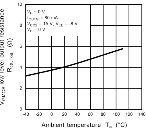
Fig. 13.3.18 R_{OUTGL} - T_a
