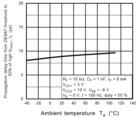
Fig. 13.3.32 t_3 - T_a
