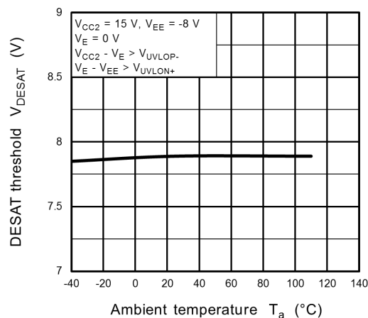
Fig. 13.3.25 V_{DESAT} - T_a
