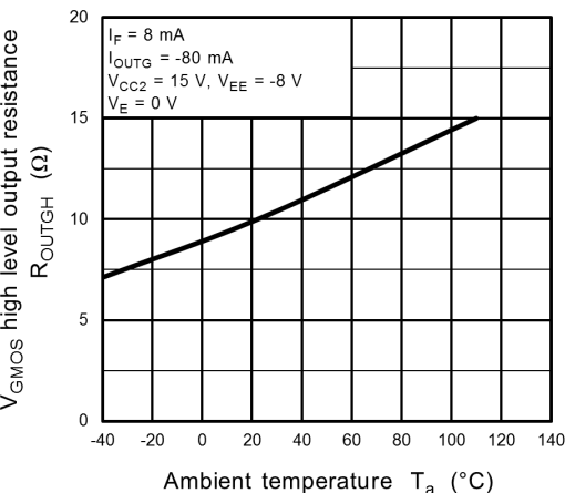
Fig. 13.3.17 R_{OUTGH} - T_a
