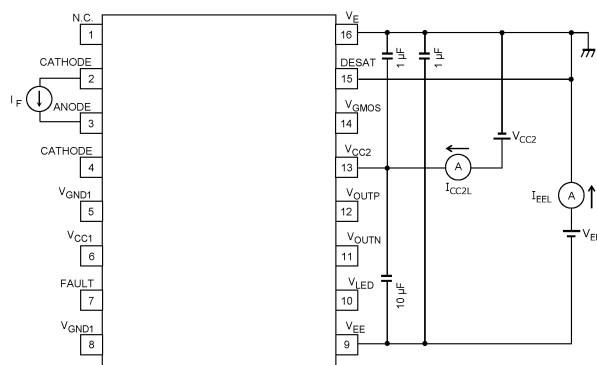
Fig. 13.1.14 I CC2L , I HEEL Test Circuit
