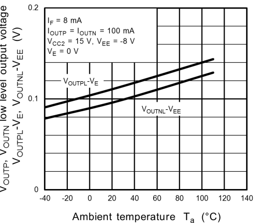
Fig. 13.3.16 V_{OUTPL} - V_E , V_{OUTNL} - V_{EE} - T_a
