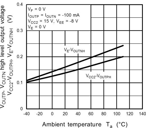
Fig. 13.3.15 V_{CC2} - V_{OUTPH} , V_E - V_{OUTNH} - T_a
