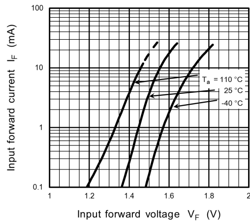
Fig. 13.3.1 I_F - V_F
