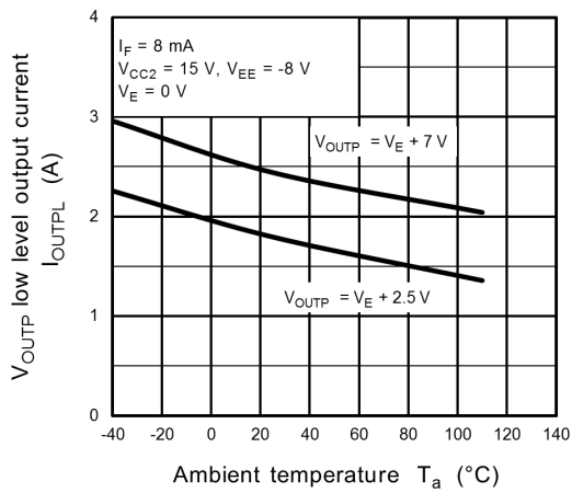
Fig. 13.3.4 I_{OUTPL} - T_a
