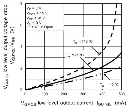
Fig. 13.3.12 (V_{OUTGL} - V_{EE}) - I_{OUTGL}
