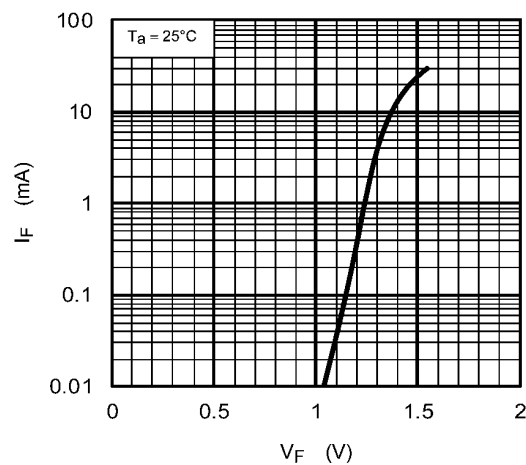
Fig. 12.3 I_F - V_F
