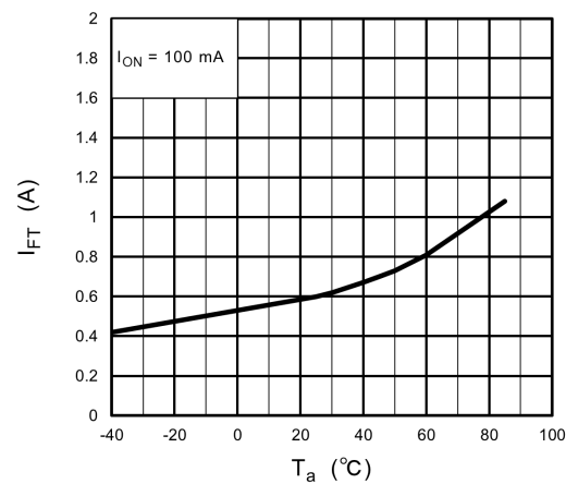
Fig. 12.6 I_{FT} - T_a
