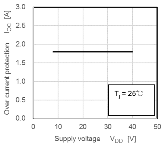
I_{OC} - V_{DD}
