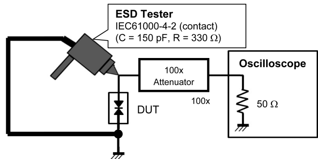
Fig. 6.1.3 IEC61000-4-2 (Contact)
