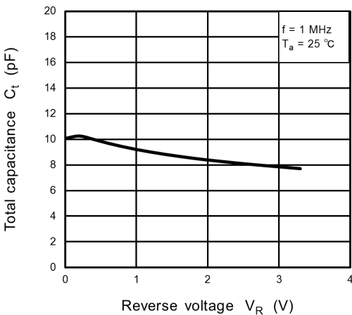
Fig. 9.3 C_t - V_R
