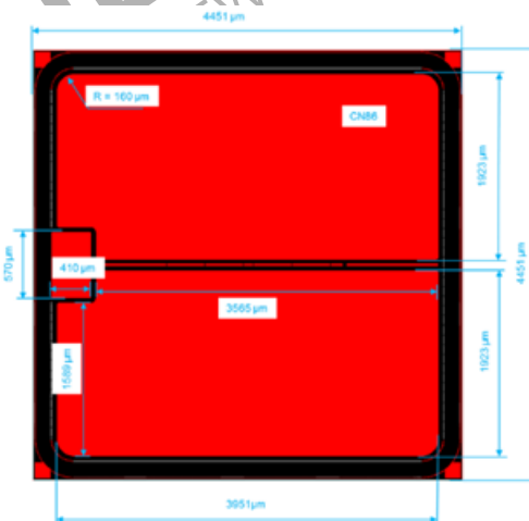
DIE OUTLINE
