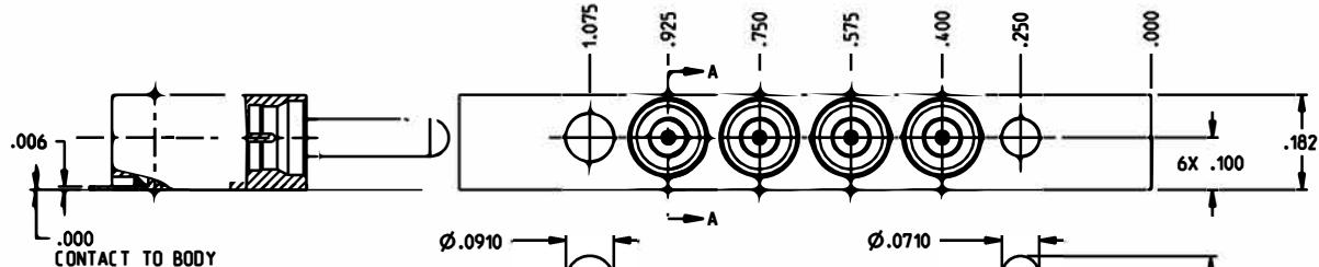
4X SECTION A-A
