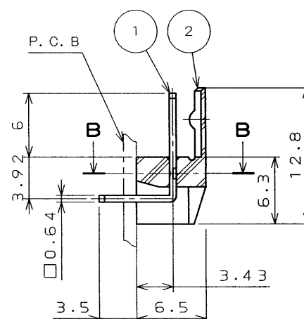
断面 A—A
