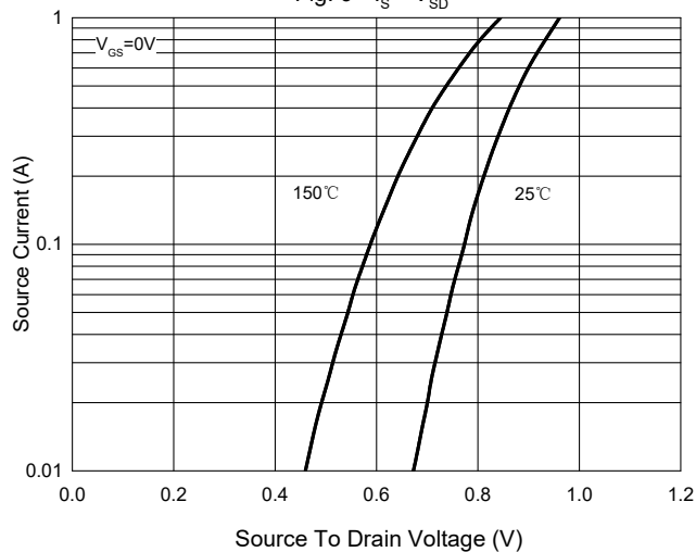
Fig. 9 - I_S - V_{SD}
