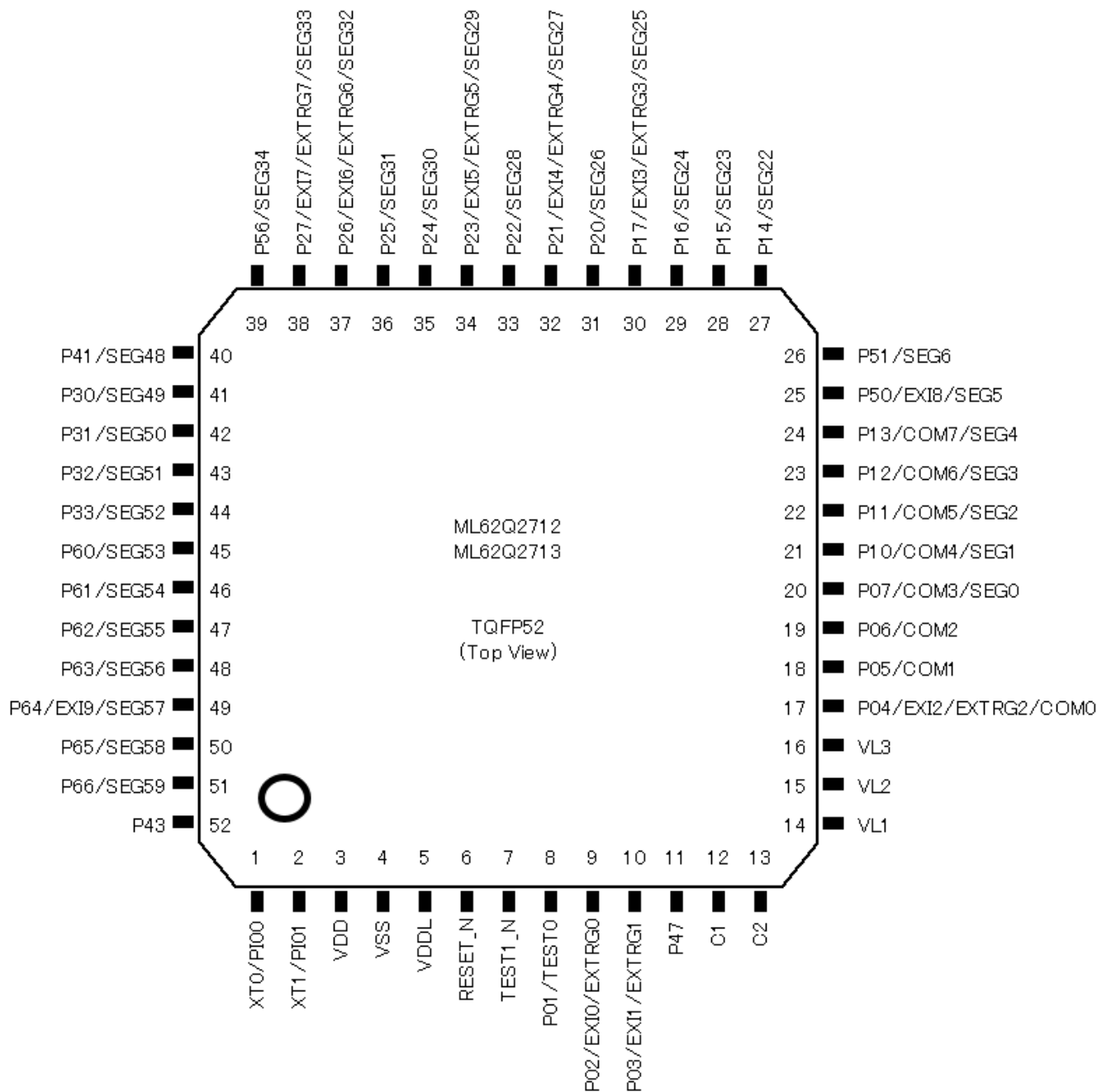
Fig.3-5 52 pin TQFP
