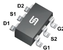
SOT-26
