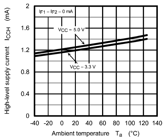
Fig. 12.2.8 I_{CCH} - T_a
