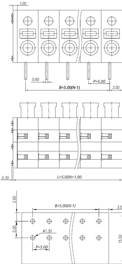
P.C.B. LAYOUT
