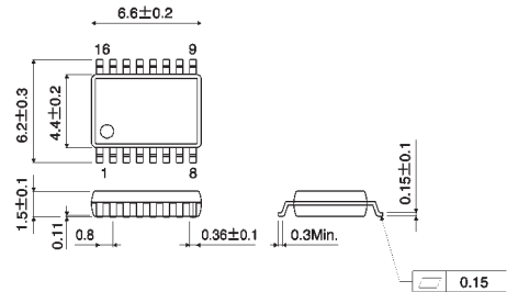
SSOP-A16
