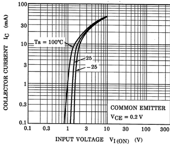
Fig. 14.1 Q1 I_C - V_{I(ON)}
