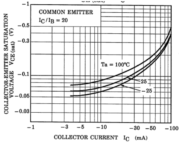
Fig. 14.8 Q2 V_{CE(sat)}-I_C
