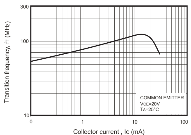
Fig.6- f_T - I_C
