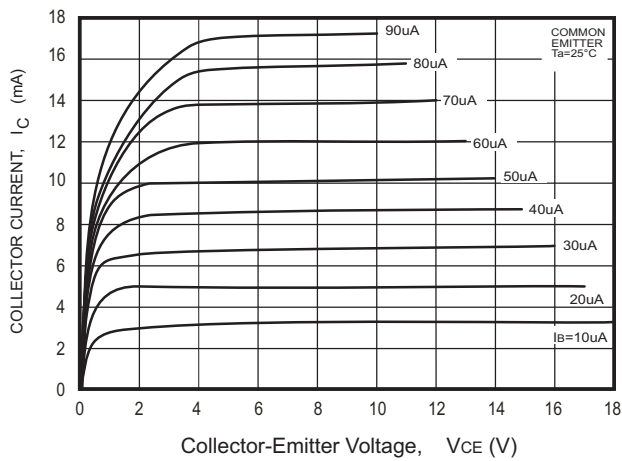
Fig.1- I_C - V_{CE}
