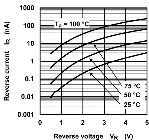
Fig. 7.2 I_R - V_R
