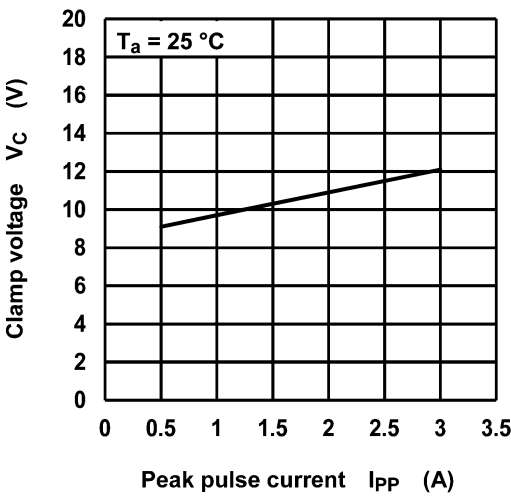
Fig. 8.1 V_C - I_{PP}
