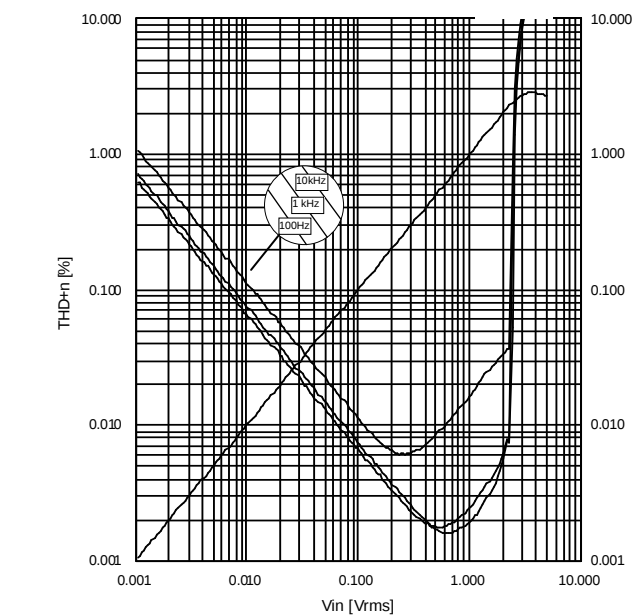
Figure 6. THD+N, Vo vs. Vin
