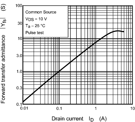
Fig. 9.8 |Y_{fs}| - I_D
