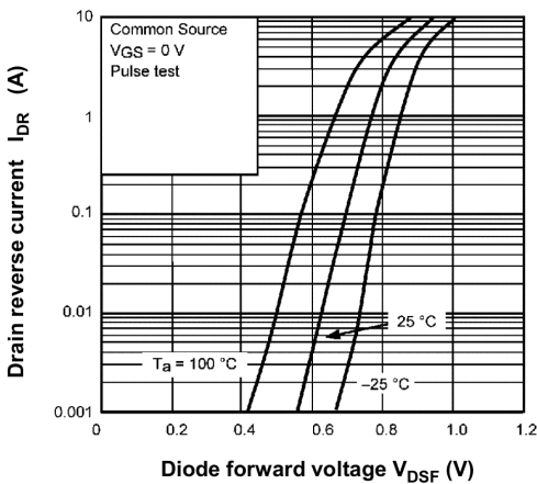
Fig. 9.9 I_{DR} - V_{DSF}
