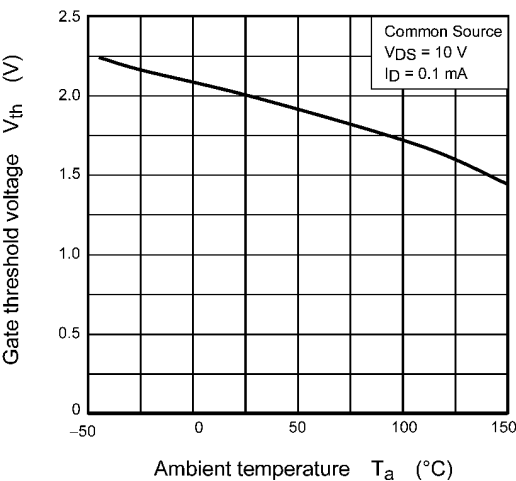
Fig. 9.7 V_{th} - T_a
