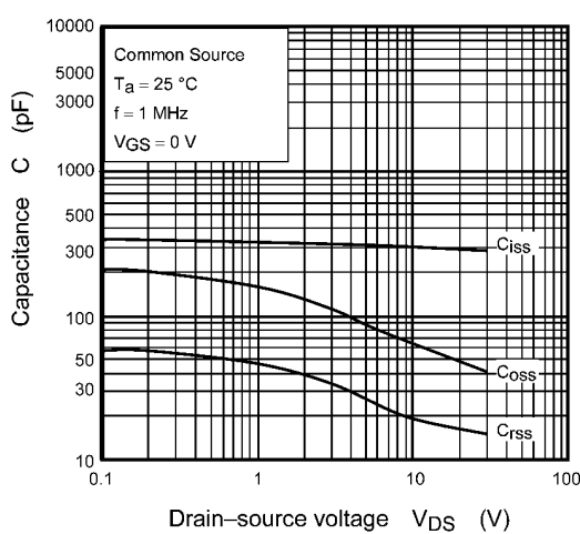
Fig. 9.10 C - V_{DS}
