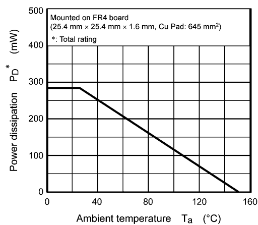
Fig. 7.14 P_D - T_a
