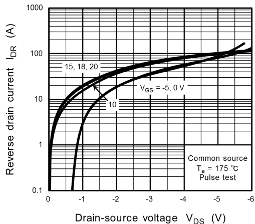
Fig. 8.10 I_{DR} - V_{DS}
