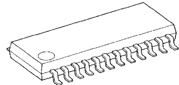
SSOP24-P-300-1.00B
