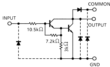
TD62004AP/AF
