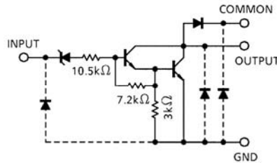
TD62002AP/AF
