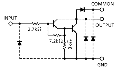
TD62003AP/AF
