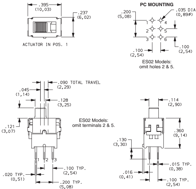
ES21MCBE DPDT
