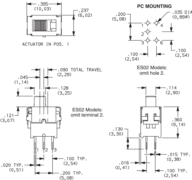
ES01MCBE SPDT
