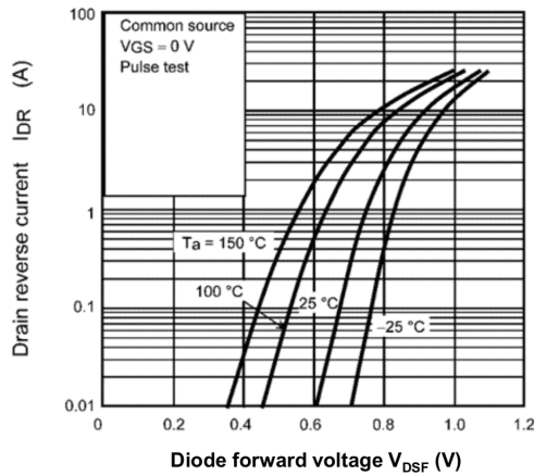
Fig. 9.7 I_{DR} - V_{DSF}
