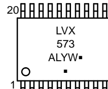
TSSOP-20
