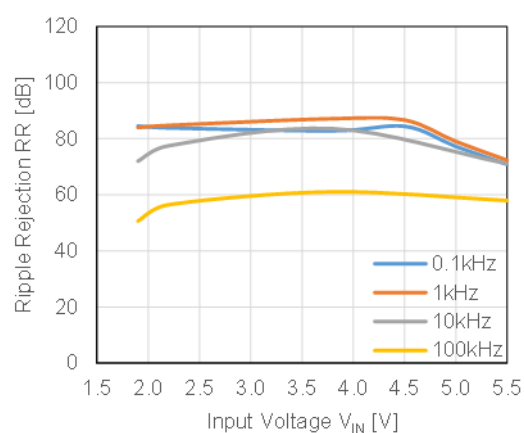
RP123x28xx, I_{OUT} = 250\text{ mA}
