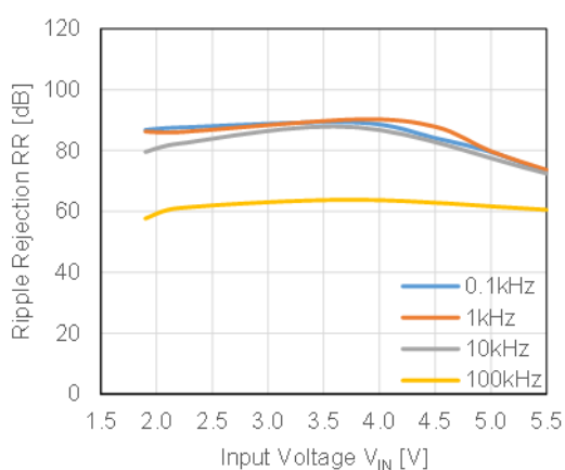
RP123x28xx, I_{OUT} = 100\text{ mA}
