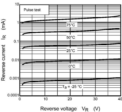
Fig. 9.2 I_R - V_R
