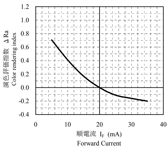
演色評価指数 — 順電流特性 Color rendering index vs. Forward Current (Tc=25 °C)
