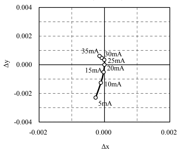
色度座標 — 順電流特性 Chromaticity coordinates vs. Forward Current (Tc=25 °C)
