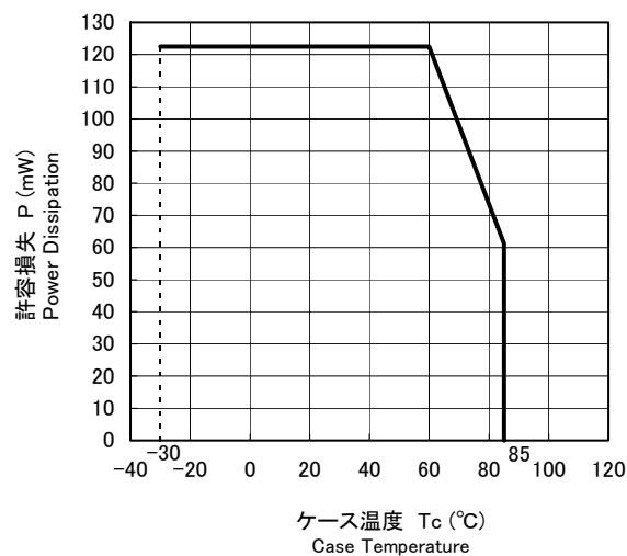
許容損失低減曲線 Power Dissipation Derating Curve
