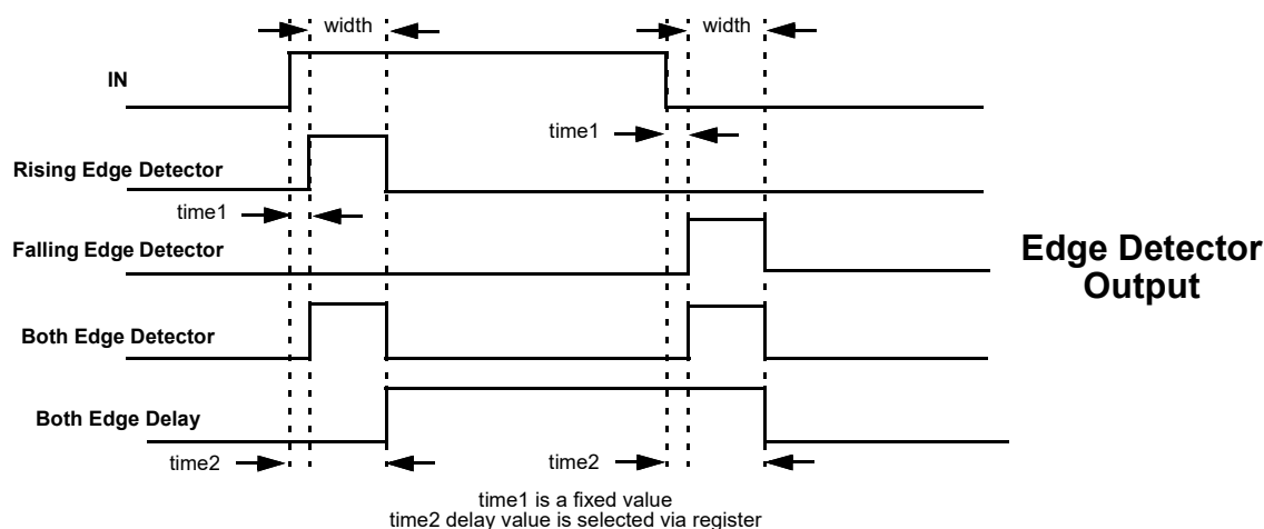
Figure 24. Edge Detector Output
