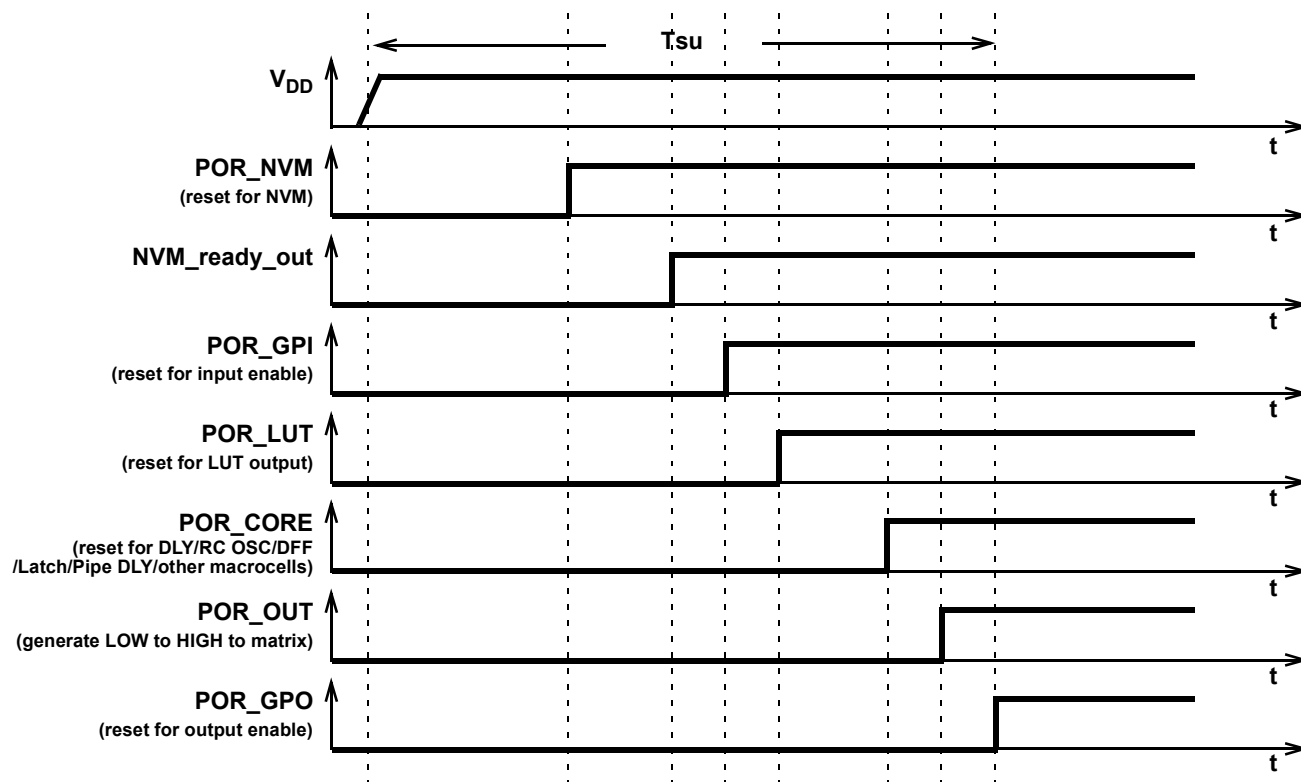
Figure 34. POR Sequence
