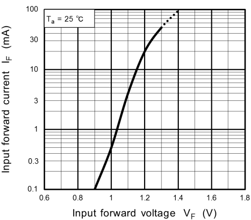
Fig. 12.4 I_F - V_F
