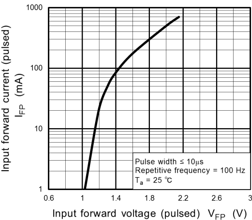
Fig. 12.6 I_{FP} - V_{FP}
