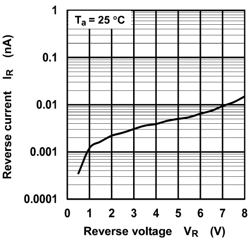
Fig. 8.2 I_R - V_R
