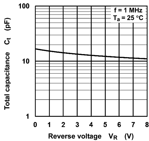
Fig. 8.3 C_t - V_R
