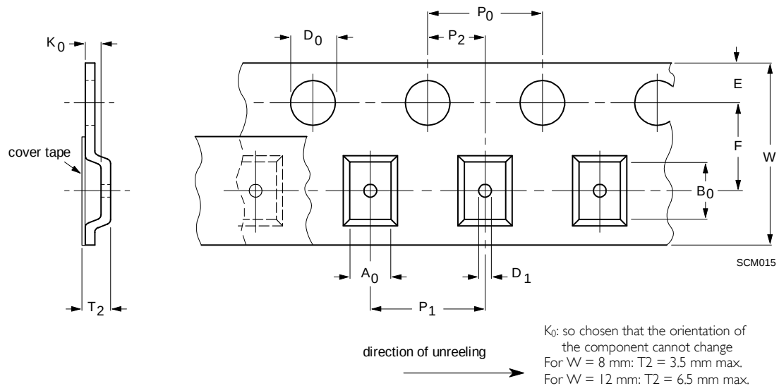
Fig. 4 Blister tape
