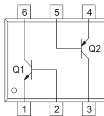
CMLT3946E CMLT3946EG*
