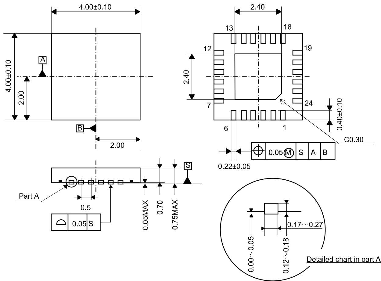
Fig. 16 Outer Dimensions
