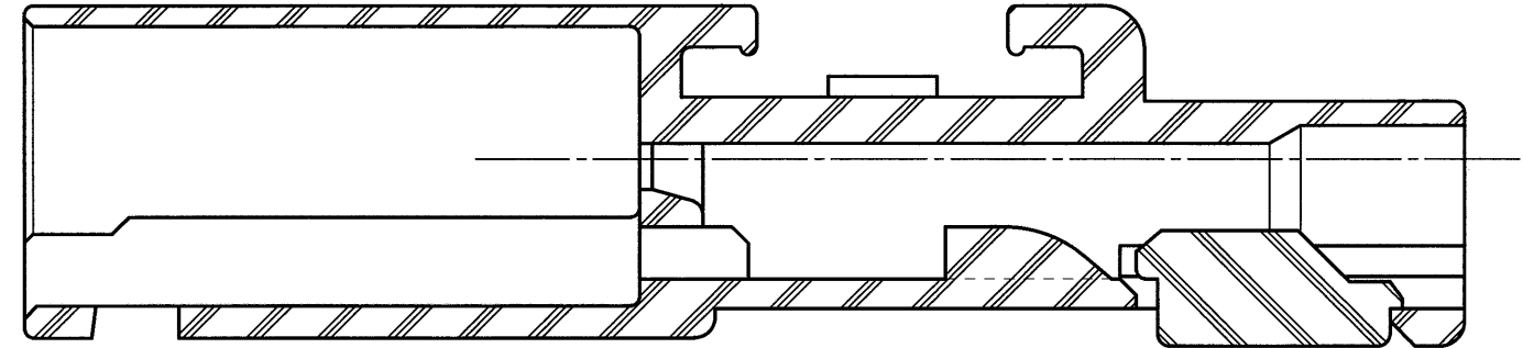
SECT. A-A (SCALE 5:1)
