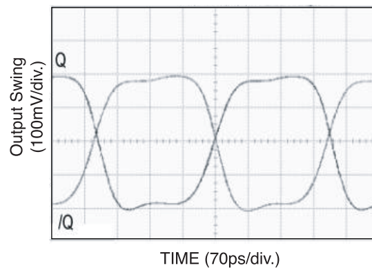
2GHz Clock
