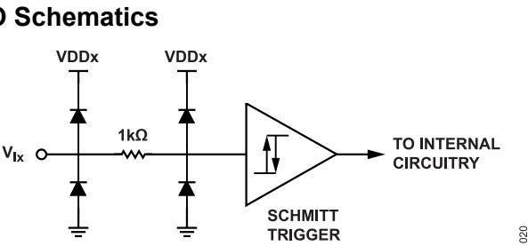
Figure 23. V IA , V IB , V IC , V ID , V IE , V IF Input Schematics
