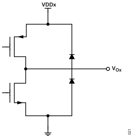
Figure 24. V OA , V OB , V OC , V OD , V OE , V OF Output Schematics
