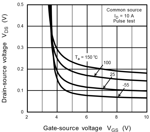
Fig. 8.3 V_{DS} - V_{GS}
