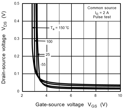
Fig. 8.5 V_{DS} - V_{GS}
