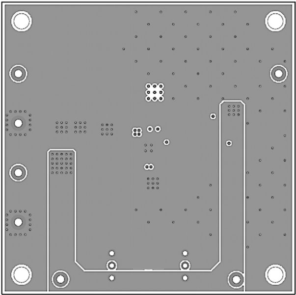
Middle 2 Layer
