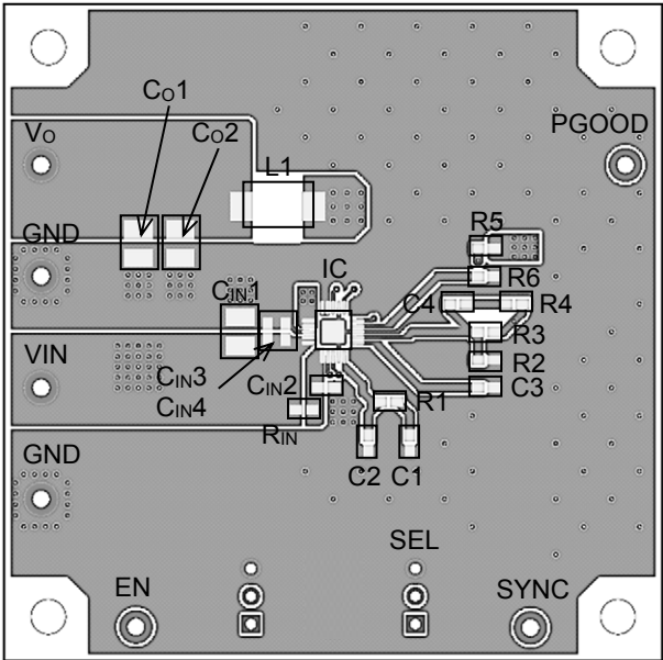
TOP Layer
