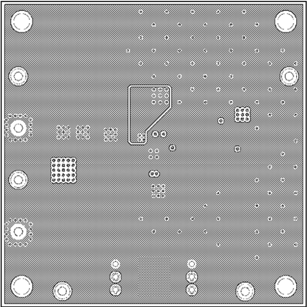
Middle 1 Layer
