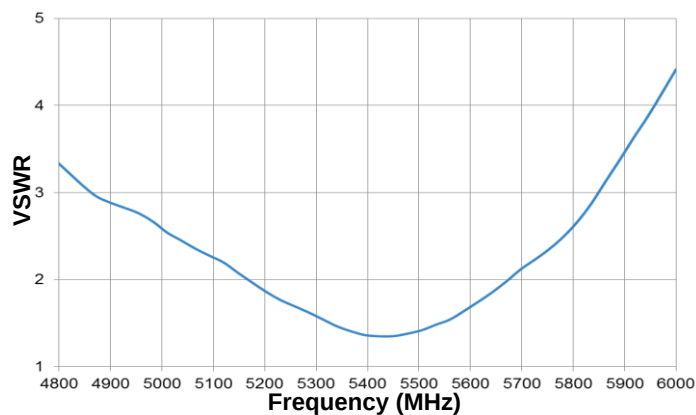
5 GHz VSWR
