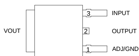
TO252-2 (5)
